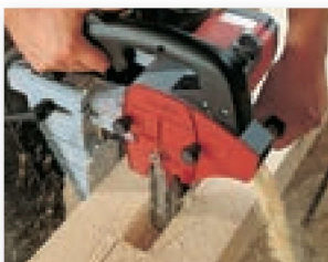
Dlaby s LS 103 Ec s různými rozměry do 100 mm.
