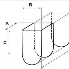
Rozměry frézovacích řetězů Příklad: 28 x 40 x 100 mm Šířka frézovacího řetěze A: 28 mm Šířka otvoru B: 40 mm Hloubka dlabu C: 100 mm
